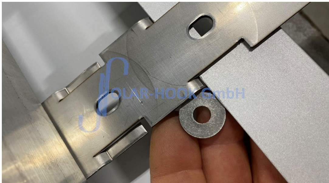
Abb. 4/SOLAR-HOOK Befestigungsbügel am Modulrahmen mit Unterlegscheibe
