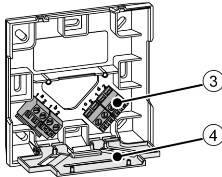
Klemmenkontakte
